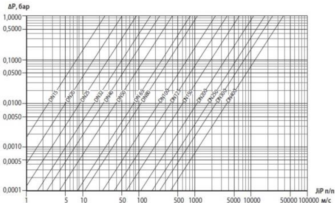
Диаграмма потерь давления крана шарового типа JiP Full Bore.
