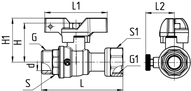
Рисунок 2 – Габаритные размеры крана.
