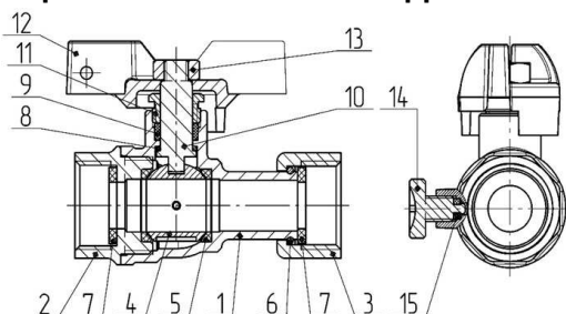
Рисунок 1 – Конструкция шарового крана
