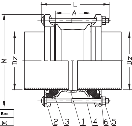
Схема монтажа
