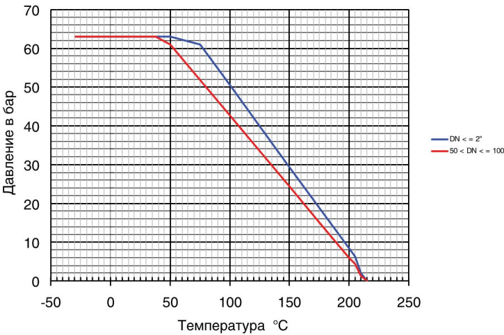
ФИК ЗАВИСИМОСТИ РАБОЧЕГО ДАВЛЕНИЯ И ТЕМПЕРАТУРЫ
