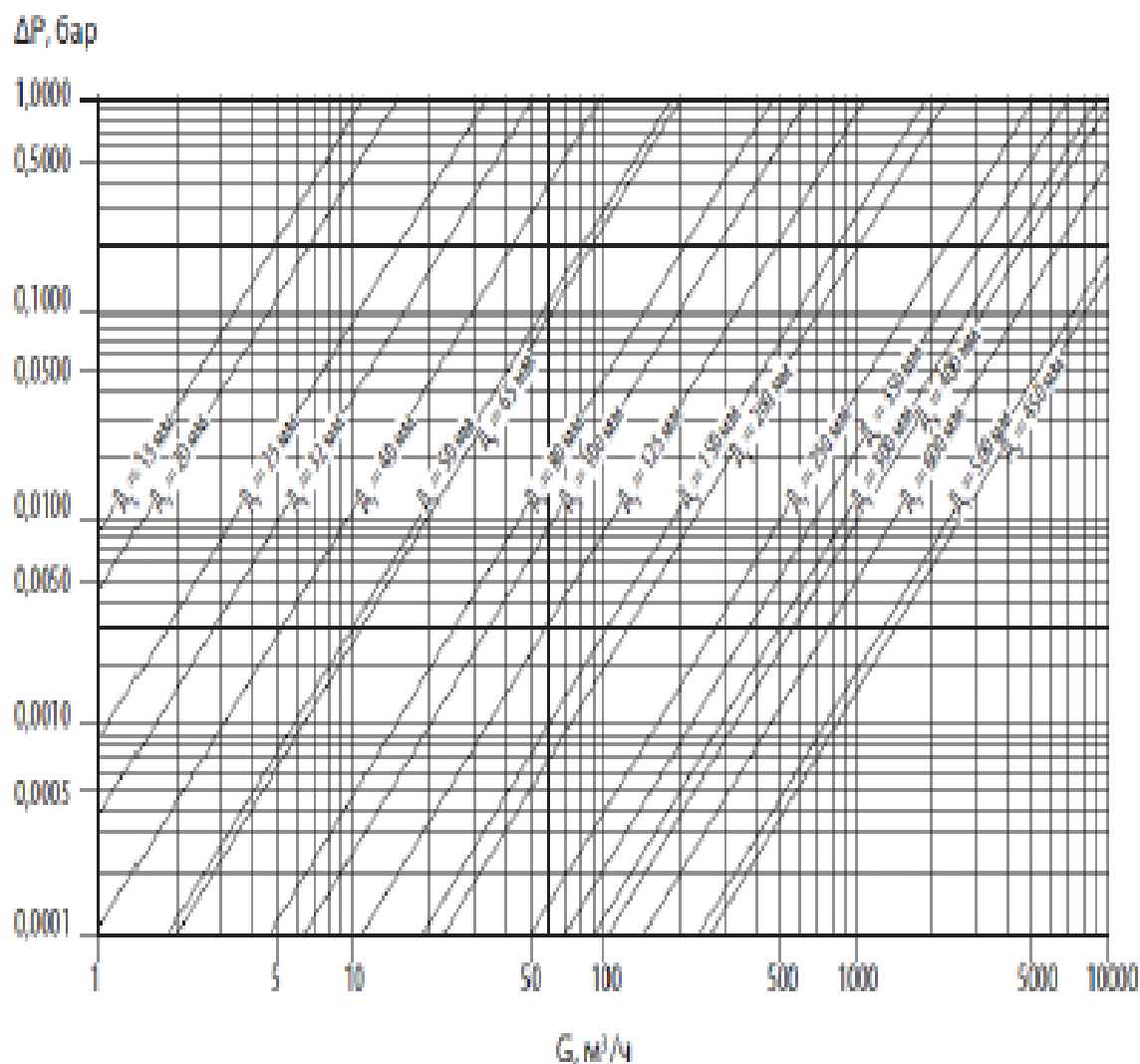
Диаграмма потерь давления крана шарового модификации JiP Premium
