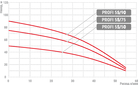
4.2. Расходно-напорные характеристики отражены на графике
