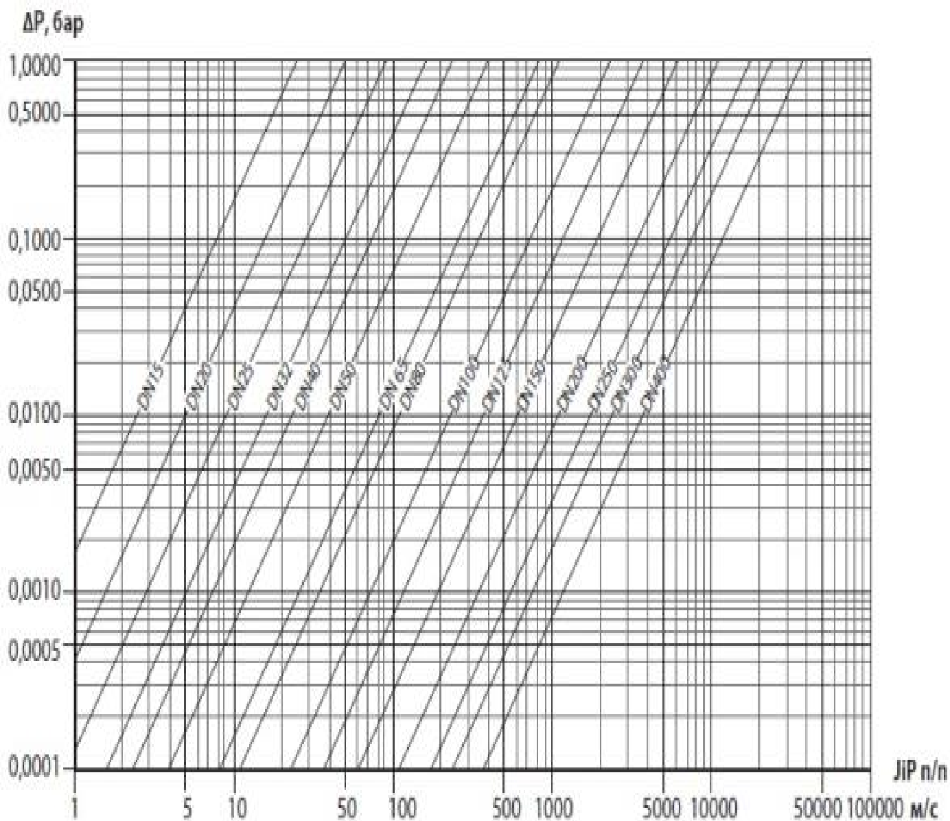
Диаграмма потерь давления крана шарового типа JiP Full Bore.
