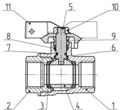
Рисунок 1 – Конструкция шарового крана
