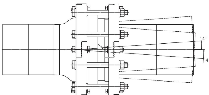
Рисунок. Допустимое отклонение трубопровода
