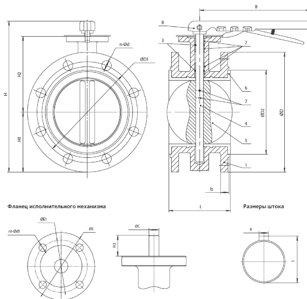
Рисунок 1. Затворы DN 50-300
