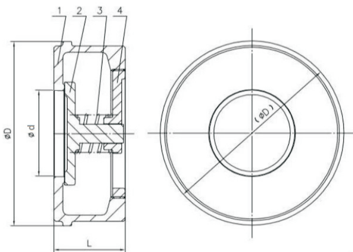
Чертеж габаритный обратного клапана тарельчатого межфланцевого ABRA-D71( размеры в таблице ниже):
