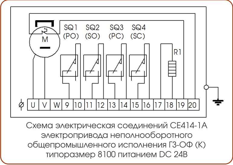
Схема электрическая соединений CE411-7A электропривода непрямого вращения общепромышленного исполнения ГЗ-ОФ (К) типоразмер 8100 питанием 3 AC 400В 50Гц
