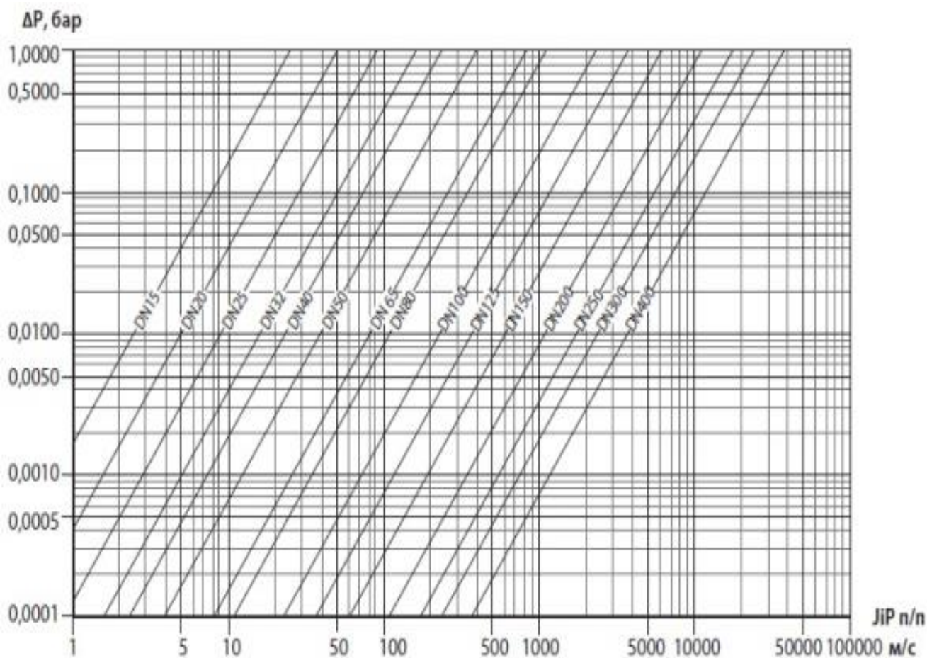
Диаграмма потерь давления крана шарового типа JiP Full Bore.
