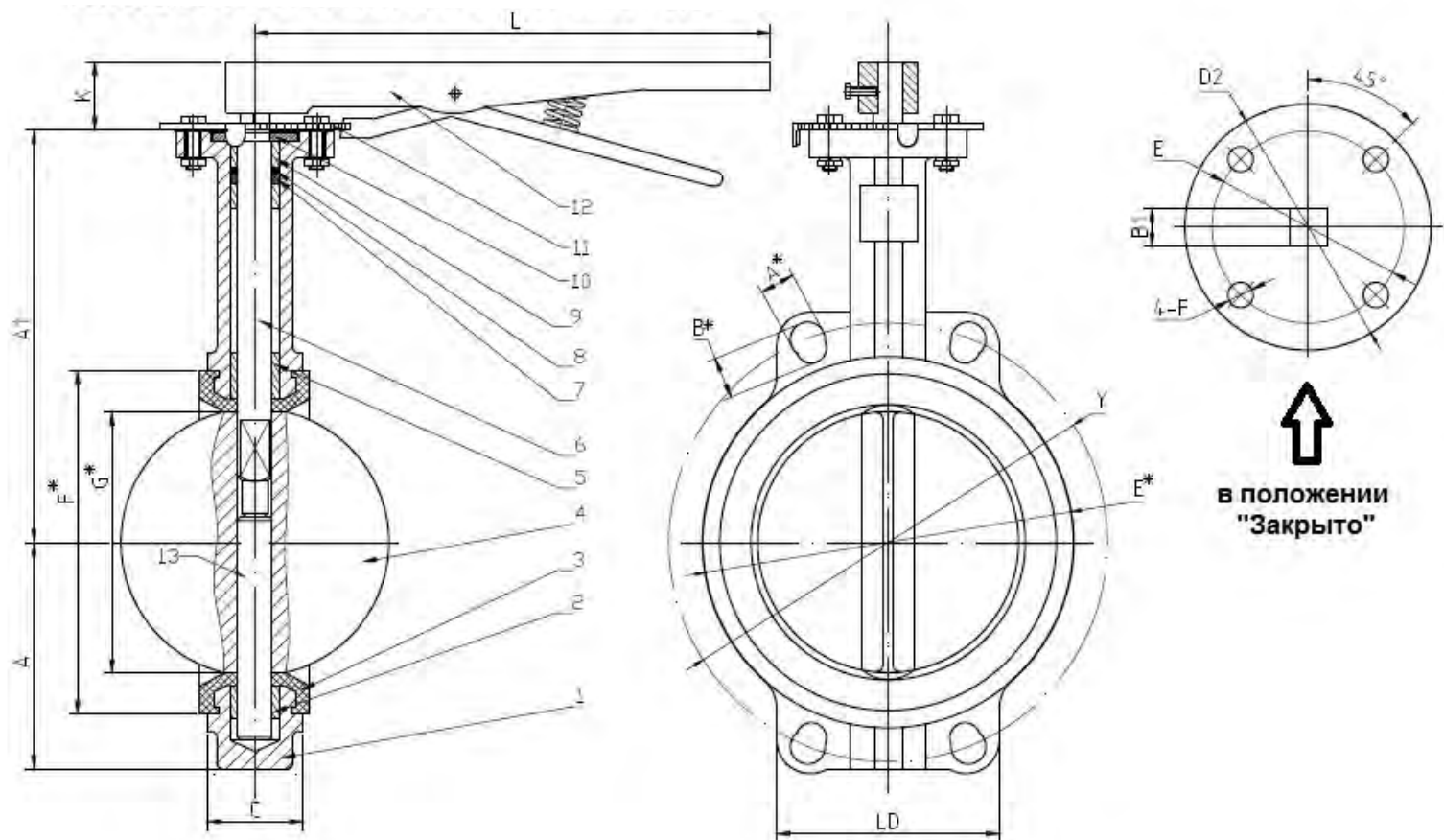
ABRA-BUV-VF866 DN100-300 PN10/16
