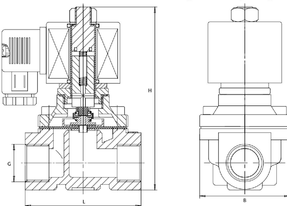
Рис.1. Клапан тип VZ
