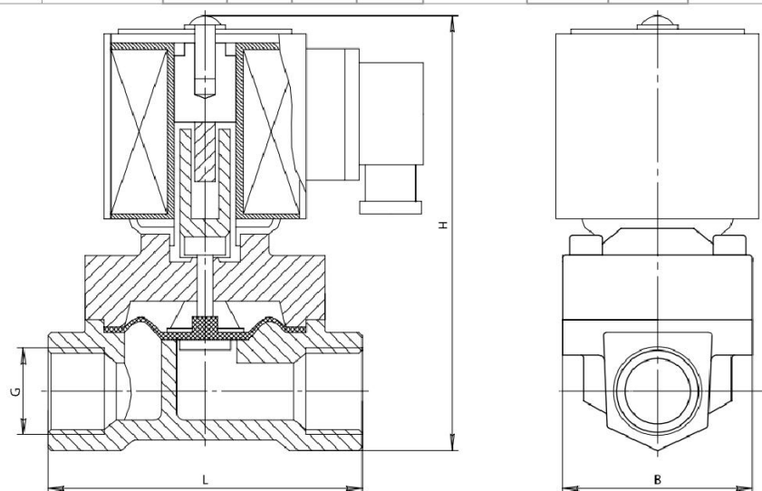
Рис. 2. Клапан тип VS
