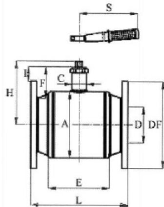
Габаритные и присоединительные размеры кранов шаровых типа JiP, фланцевые.
