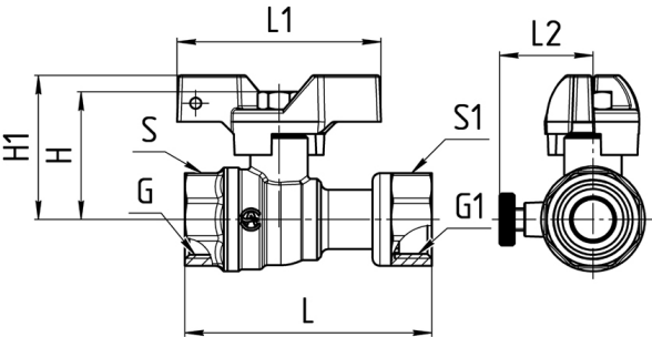
Рисунок 2 – Габаритные размеры крана.
