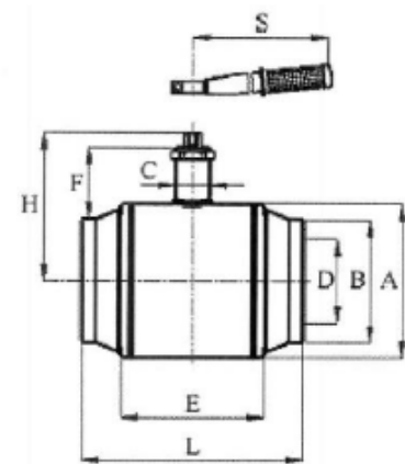
Габаритные и присоединительные размеры кранов шаровых типа JiP с рукояткой и патрубками под приварку.
