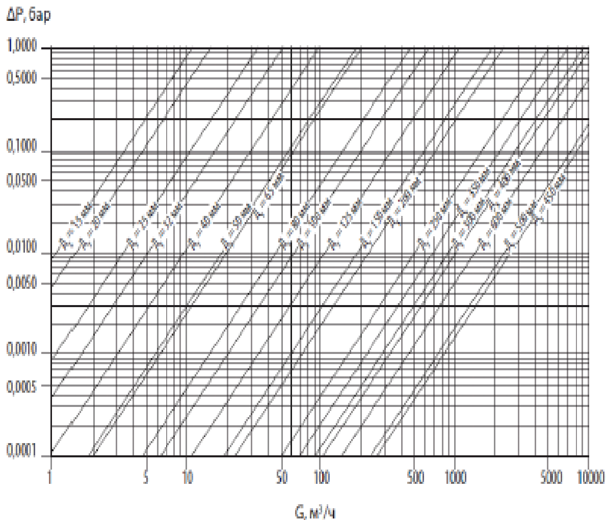
Диаграмма потерь давления крана шарового модификации JiP Premium
