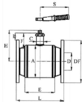
Габаритные и присоединительные размеры кранов шаровых типа JiP, фланцевые.
