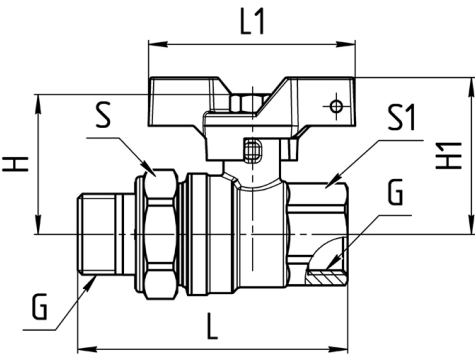
Рисунок 2 – Габаритные размеры крана.
