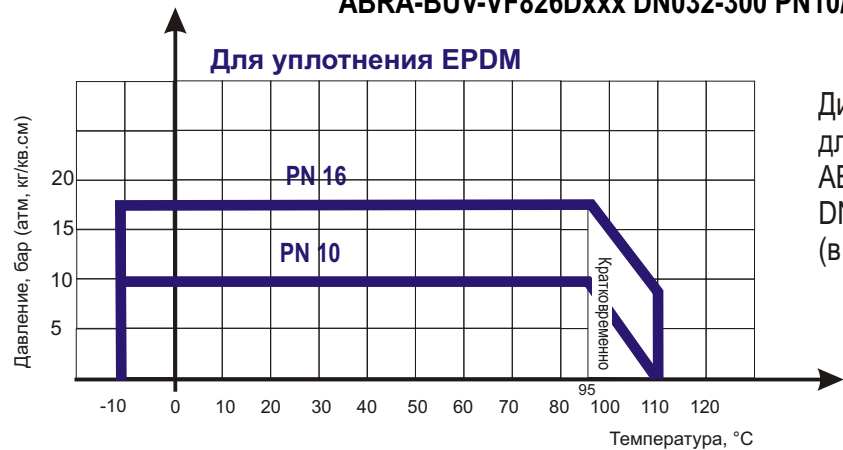
Диаграмма Давление / Температура для затвора поворотного дискового ABRA-BUV-VF826Dxxx DN032-300 PN10/16, DN350-600 PN16
